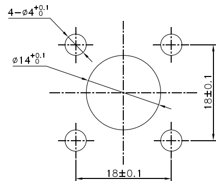
安装开孔尺寸 Mounting hole
