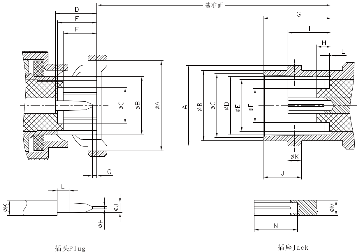
头部配合尺寸 INTERFACE MATING DIMENSIONS
