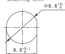
安装开孔尺寸 Mounting hole
