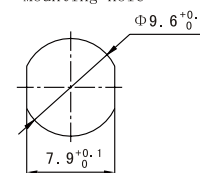
安装开孔尺寸 Mounting hole
