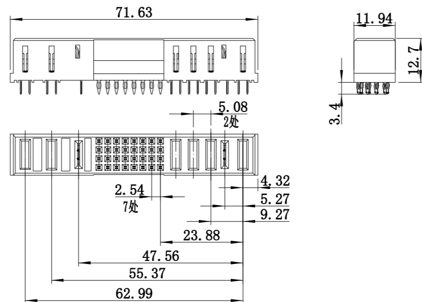
3U J0母板连接器外形尺寸 型号：C1-6450869-4
