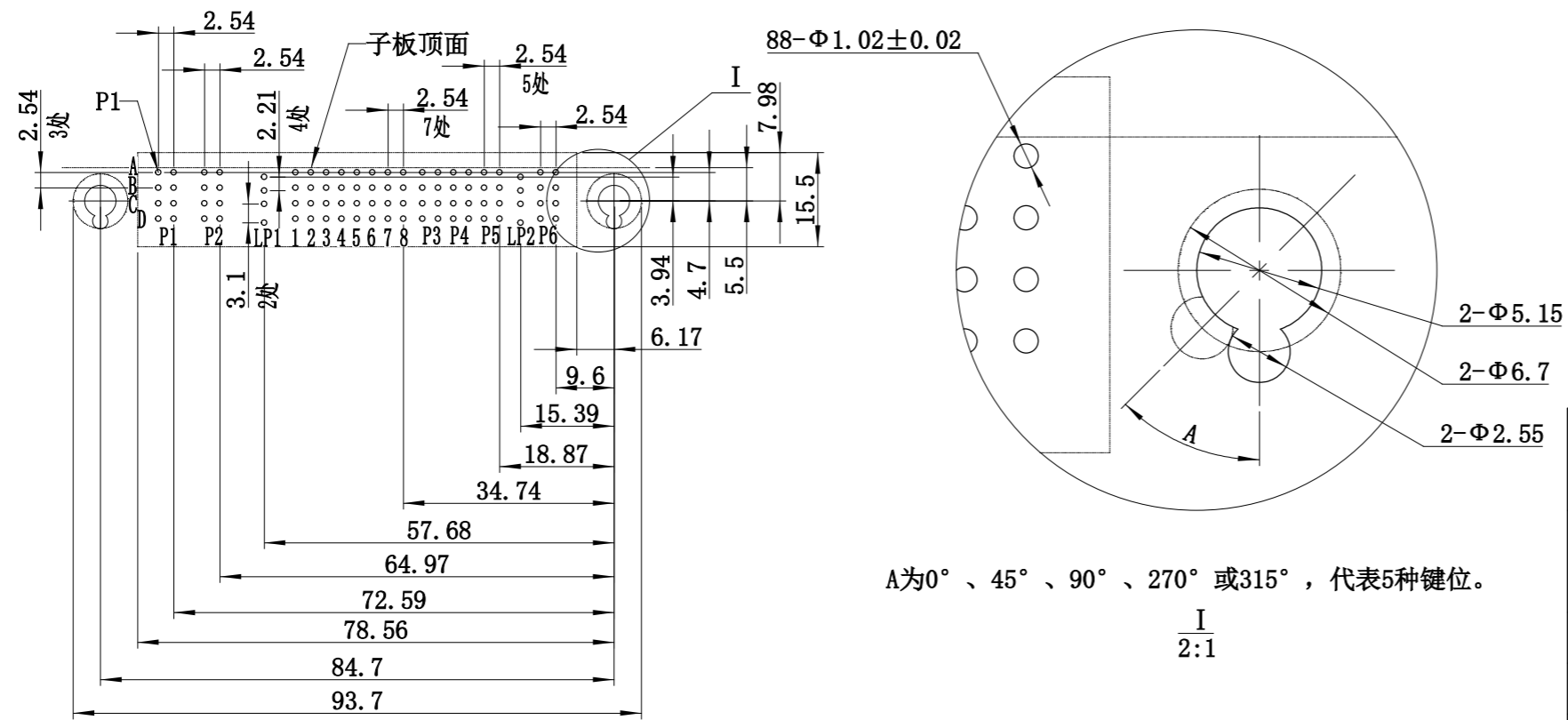
推荐PCB封装尺寸 未注公差为 \pm 0.05 \text{ mm}
