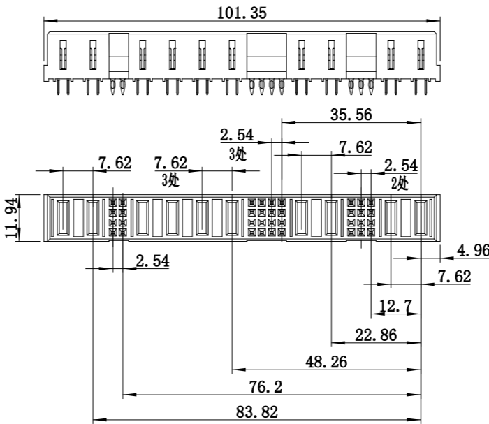
6U J1母板连接器外形尺寸 型号: C1-6450869-0
