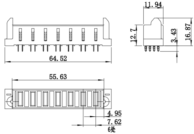
6U J0母板连接器外形尺寸 型号: C6450863-5
