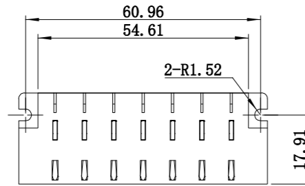
6U P0子板连接器外形尺寸 型号: C6450843-6
