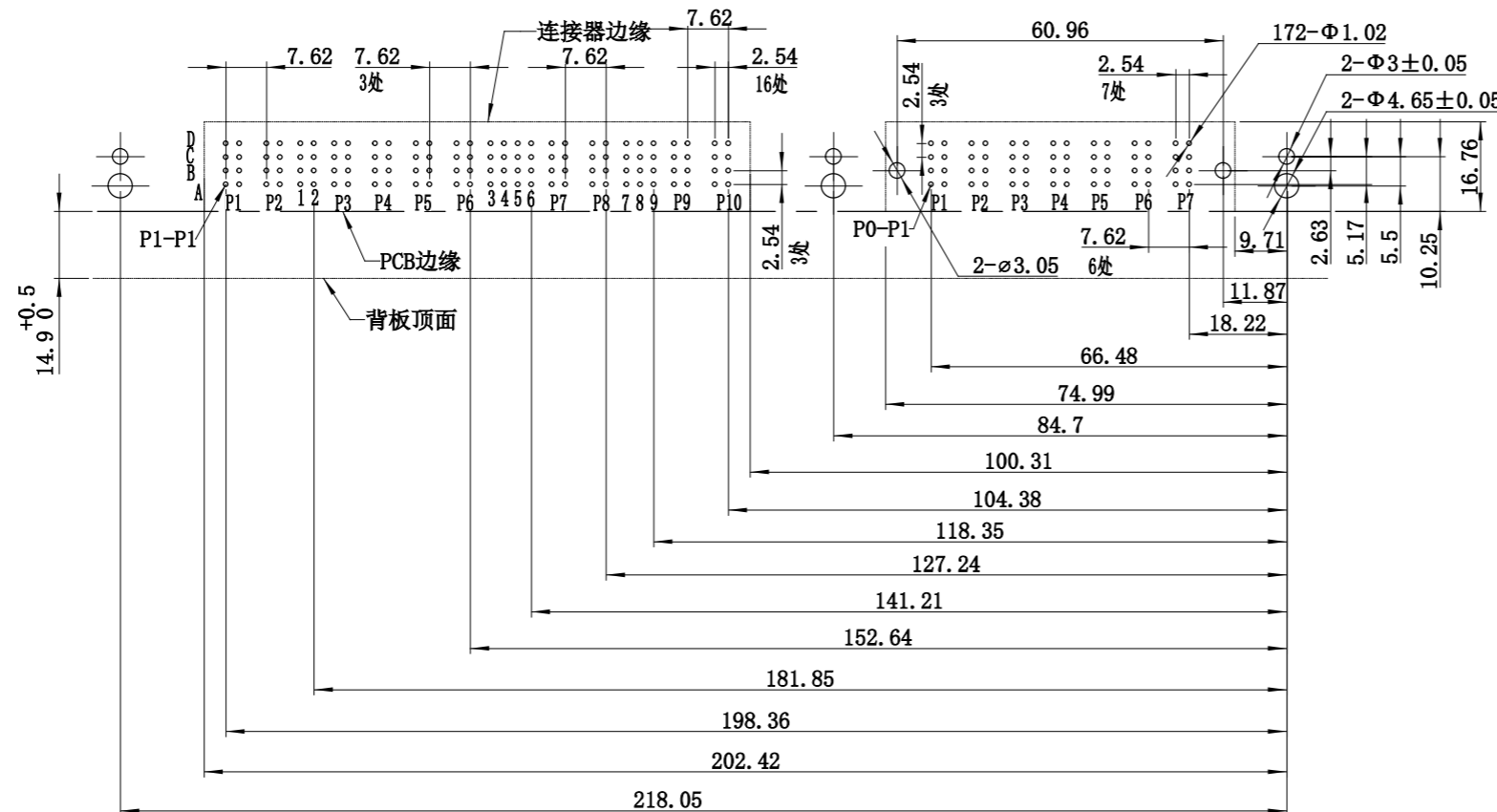
推荐PCB封装尺寸 注：P0-P1开孔尺寸型号：C6450843-6 P1-P1开孔尺寸型号：C6450849-6
