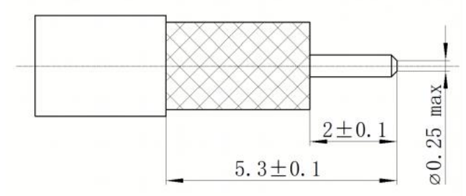
剥线尺寸
