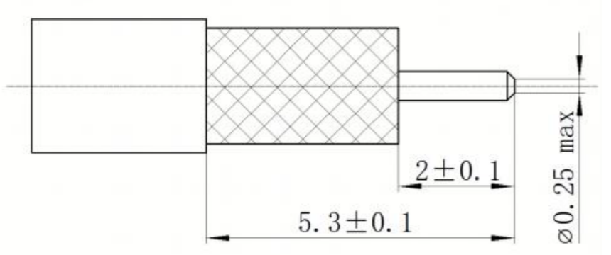
剥线尺寸
