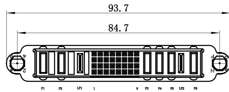
母板连接器外形尺寸 型号：VPXD-Z8A8
