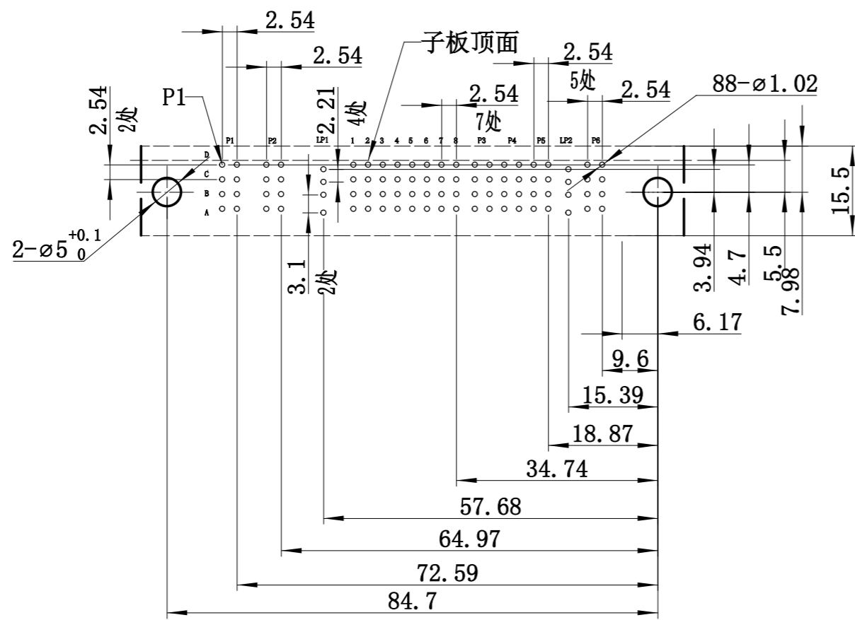
推荐PCB封装尺寸 未注公差为±0.05mm
